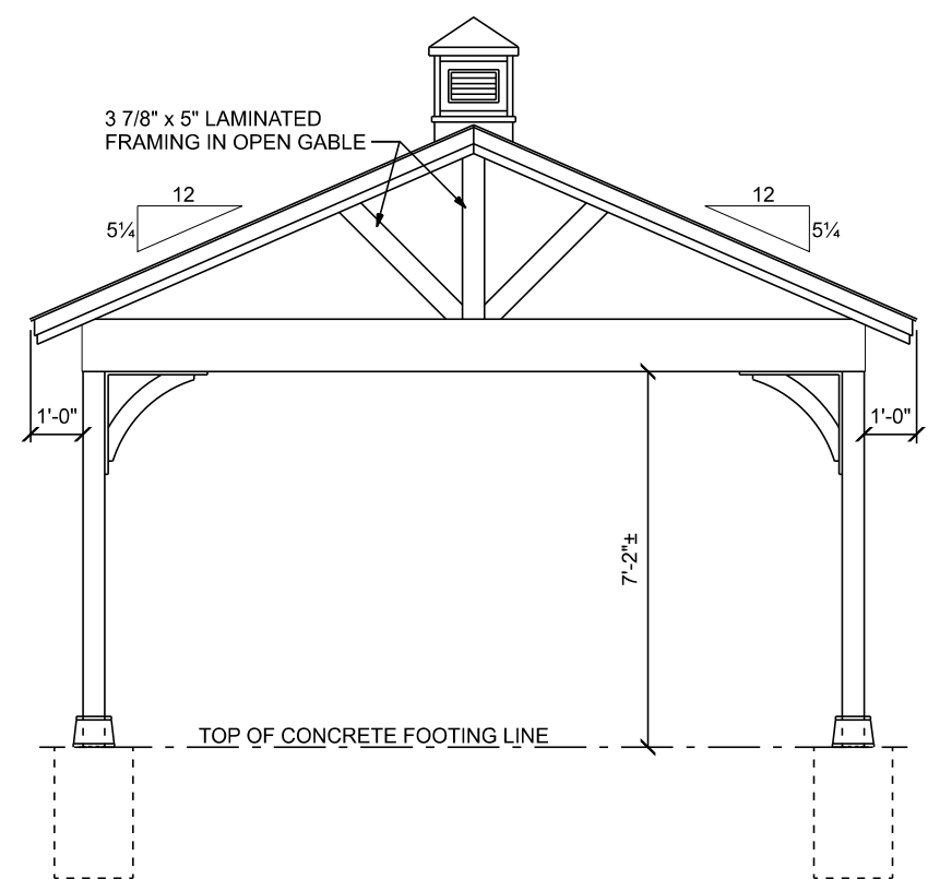
END ELEVATION
